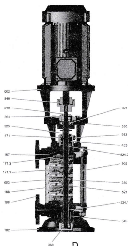
نقشه برشی الکترو پمپ
